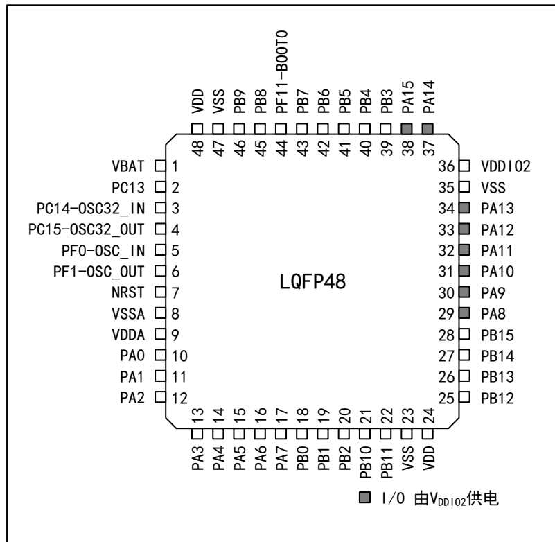
图 3 APM32F091xBxCTx 系列 LQFP48 引脚分布图
